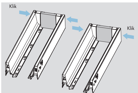
Montaža hrbtišča
