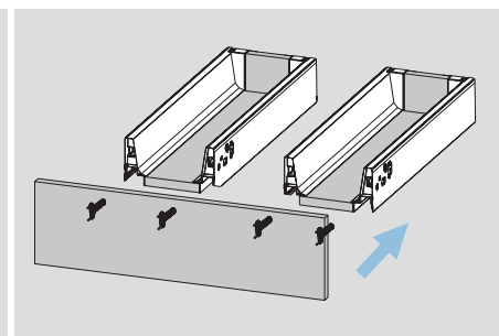
Montaža ličnice
